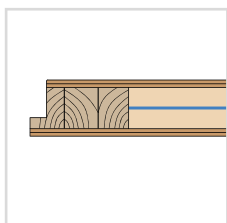
46 mm VARČIA sutvirtinta plieniniu profiliuočiu
