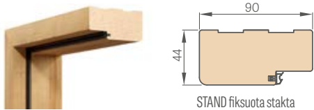
STAND fiksuota stakta
