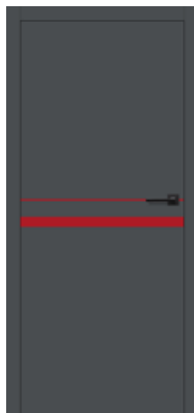
intarsija LUX 619 papildomas mokestis 76,20 €* / 92,20 €**
